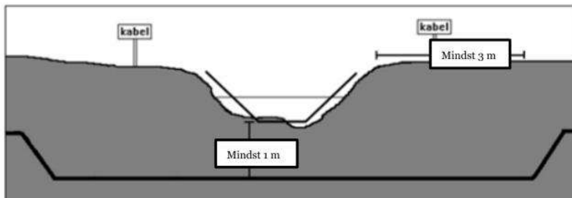
Figur 2: Korrekt ledningsføring
